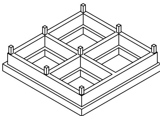
a) LOSA DE CIMENTACION NERVADA
