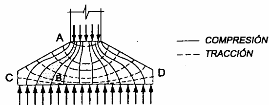
Figura 19. Red de isostáticas de una zapata aislada.
