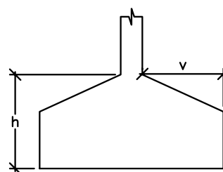
b). Zapata rígida v \leq 2h
