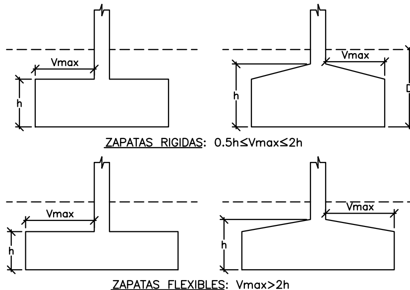
Figura 15: Clasificación de las zapatas según EHE.
